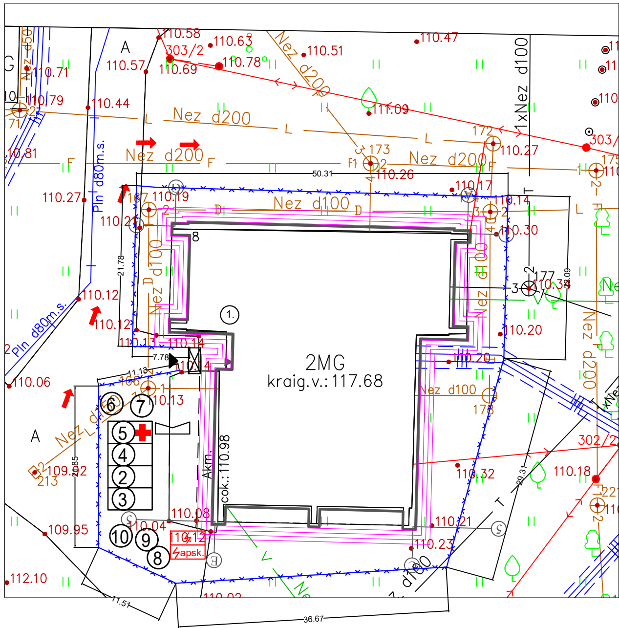
STATYBVIETĖS PLANAS M1:500
